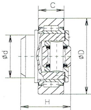
Kombirolle einstellbar mit Distanzscheiben
